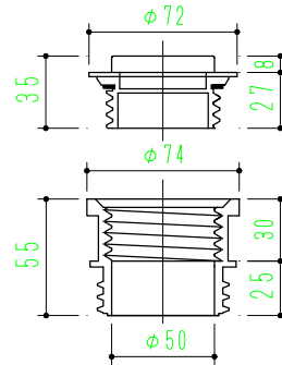
止水ボルト詳細
